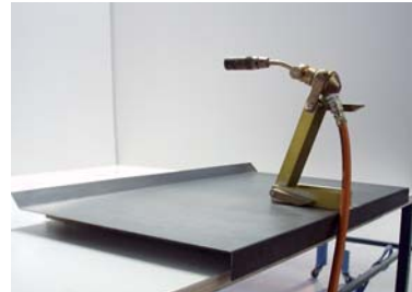
38 105 10 Arbeitsplatte für 38 102 40 Working table for 38 102 40 Ohne Brenner / without burner
