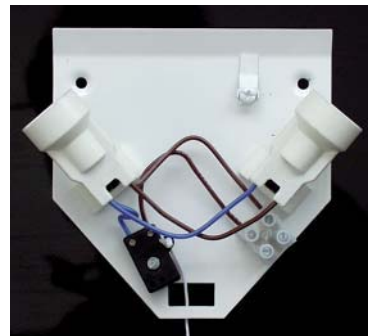
20 261 02 Wandhalter, E 14, zweiflammig, mit Zugschalter Wall fixture, E 14, 2 - light, with pull switch
